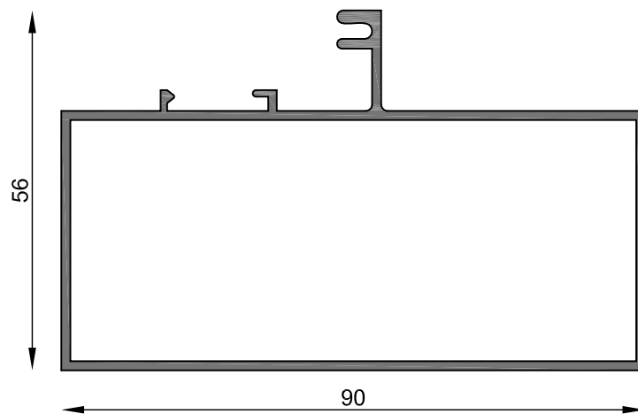
MT-0711 Paño fijo tubular (90 x 40 mm) Peso estimado: 1.102 Kg/m Largo STD: 6150 mm
