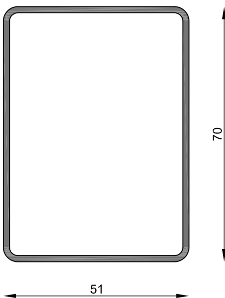
MT-5401 Empalme de columna LUV 974 Peso estimado: 1.061 Kg/m Largo STD: 6000 mm
