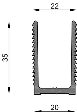
MT-0479 "U" de armado Peso estimado: 0.489 Kg/m Largo STD: 6030 mm
