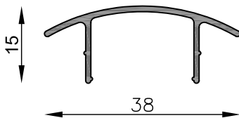
MT-0894 Tapa Peso estimado: 0.189 Kg/m Largo STD: 6030 mm
