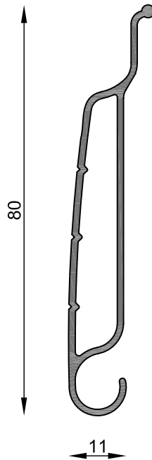
MT-2853 Tablilla cortina de enrollar Peso estimado: 0.532 Kg/m Largo STD: 6030 mm
