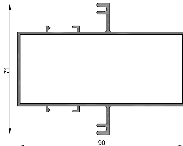
MT-0700 Travesaño tubular paño fijo Peso estimado: 1.242 Kg/m Largo STD: 6030 mm
