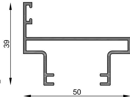
MT-0893 Marco puerta tabique Peso estimado: 0.513 Kg/m Largo STD: 6150 mm
