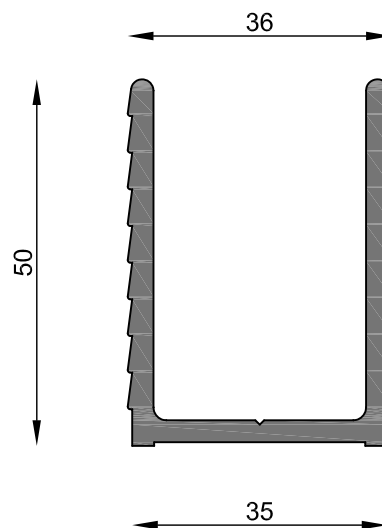
MT-2457 "U" de armado Peso estimado: 1.094 Kg/m Largo STD: 6030 mm
