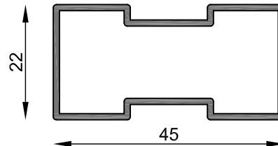
MT-0194 Travesaño tabiquería tubular Peso estimado: 0.459 Kg/m Largo STD: 6030 mm
