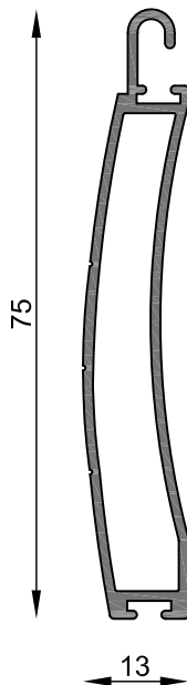
MT-1982 Zócalo de cortina Peso estimado: 0.554 Kg/m Largo STD: 6030 mm
