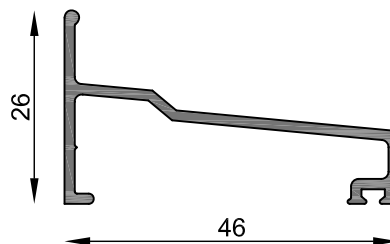
MT-1349 Umbral sanitario cubre bañera Peso estimado: 0.348 Kg/m Largo STD: 6030 mm
