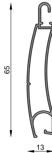
MT-0991 Tablilla de Cortina Peso estimado: 0.424 Kg/m Largo STD: 6030 mm
