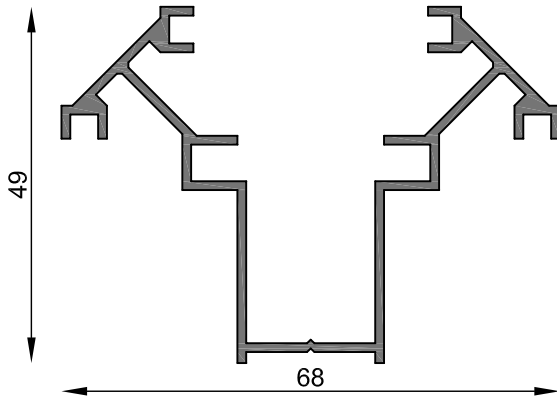
MT-1391 Columna tabique divisorio Peso estimado: 0.726 Kg/m Largo STD: 6030 mm
