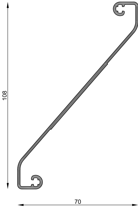
MT-0650 Parasol fijo Peso estimado: 0.780 Kg/m Largo STD: 6030 mm
