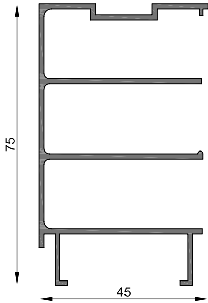
MT-0190 Zócalo tabiquería tubular Peso estimado: 0.996 Kg/m Largo STD: 6030 mm
