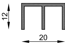
MT-1674 Dintel vitrina Peso estimado: 0.184 Kg/m Largo STD: 6030 mm
