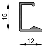
MT-0192 Contravidrio corto Peso estimado: 0.111 Kg/m Largo STD: 6030 mm
