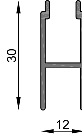
MT-1012 Umbral vitrina Peso estimado: 0.240 Kg/m Largo STD: 6030 mm
