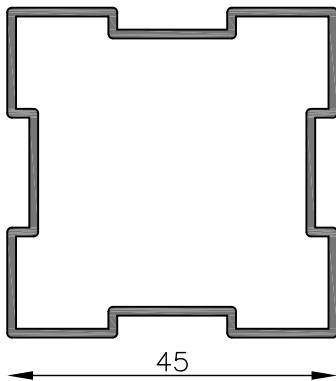
MT-0195 Columna tabiquería tubular Peso estimado: 0.640 Kg/m Largo STD: 6030 mm
