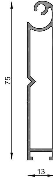
MT-2852 Zocalo cortina de enrollar Peso estimado: 0.643 Kg/m Largo STD: 6030 mm
