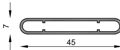
MT-0802 Tablilla celosia Peso estimado: 0.302 Kg/m Largo STD: 6030 mm
