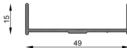
MT-1350 Jamba cubre bañera Peso estimado: 0.292 Kg/m Largo STD: 6030 mm
