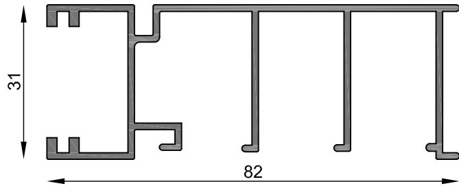
MT-2789 Zócalo Peso estimado: 0.921 Kg/m Largo STD: 6030 mm
