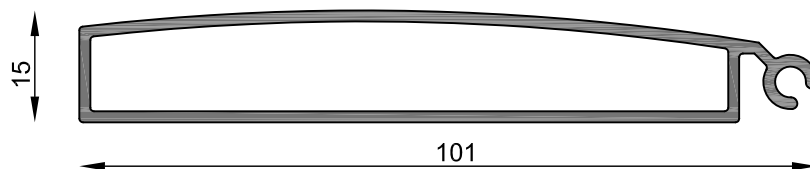
MT-2700 Zócalo cortina regulable Peso estimado: 0.894 Kg/m Largo STD: 6030 mm
