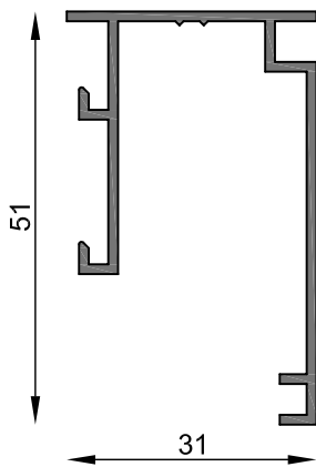
MT-1395 Dintel tabique divisorio Peso estimado: 0.440 Kg/m Largo STD: 6030 mm
