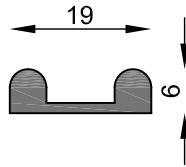
MT-1089 Riel vitrina Peso estimado: 0.184 Kg/m Largo STD: 6030 mm
