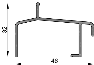
MT-0169 Umbral cubre bañera Peso estimado: 0.386 Kg/m Largo STD: 6030 mm
