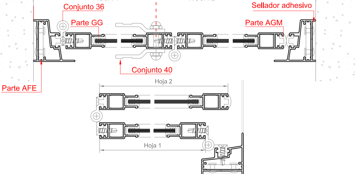
Dimensiones de corte de perfiles
