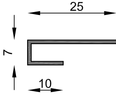
MT-1003 Perfil J 7 x 25 mm Peso estimado: 0.108 Kg/m Largo STD: 6030 mm
