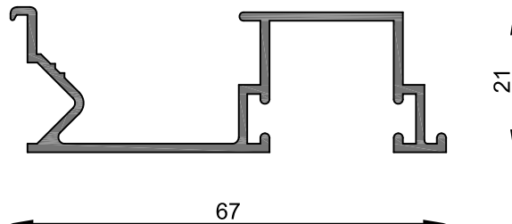
MT-0243 Guía cortina común Actual Peso estimado: 0.545 Kg/m Largo STD: 6030 mm
