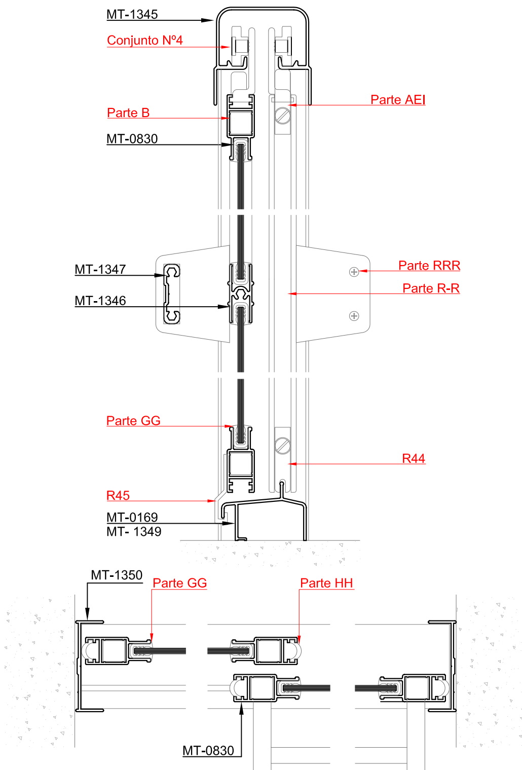
Dimensiones de corte de perfiles
