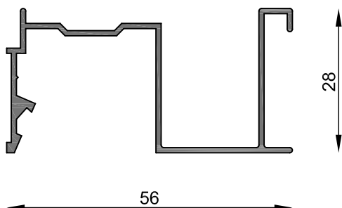
MT-0920 Guía cortina común Clásica Peso estimado: 0.419 Kg/m Largo STD: 6030 mm
