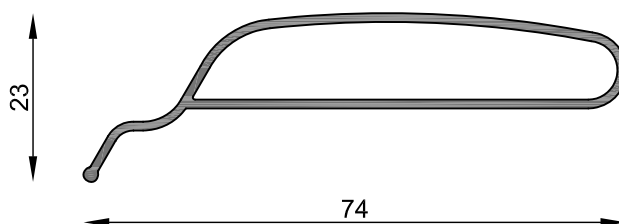
MT-2702 Tablilla cortina regulable Peso estimado: 0.481 Kg/m Largo STD: 6030 mm
