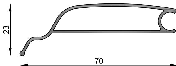
MT-2701 Primera tablilla cortina regulable Peso estimado: 0.475 Kg/m Largo STD: 6030 mm
