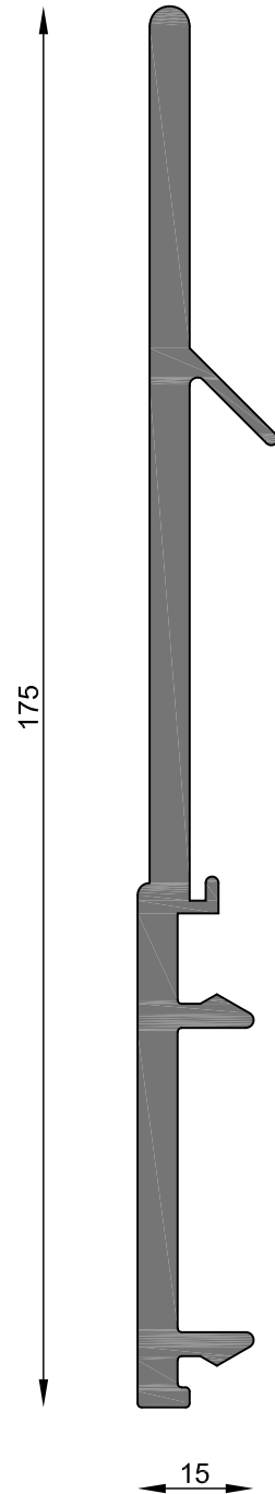
MT-5253 Presilla de cielorraso PRE 954 Peso estimado: 2.633 Kg/m Largo STD: 5500 mm
