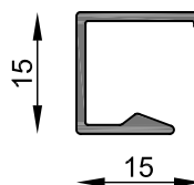
MT-0193 Contravidrio tabiquería tubular Peso estimado: 0.135 Kg/m Largo STD: 6030 mm
