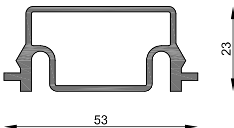
MT-5400 Presilla de revestimiento PRE 953 Peso estimado: 0.732 Kg/m Largo STD: 6000 mm
