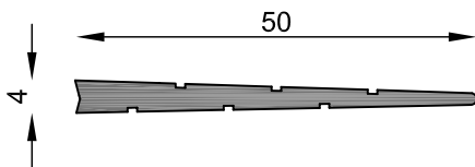
MT-5615 Cuña para escuadra CON-405/403 Peso estimado: 0.359 Kg/m Largo STD: 6030 mm
