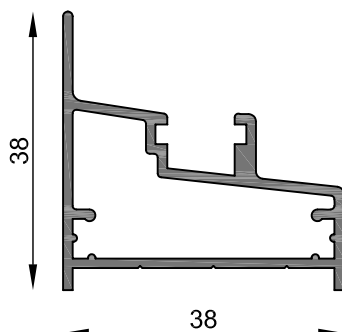
MT-0188 Marco cubre duchador Peso estimado: 0.551 Kg/m Largo STD: 6150 mm
