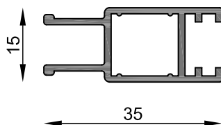
MT-0830 Hoja de mampara de baño Peso estimado: 0.346 Kg/m Largo STD: 6030 mm
