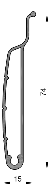
MT-1267 Tablilla cortina regulable Peso estimado: 0.510 Kg/m Largo STD: 6030 mm
