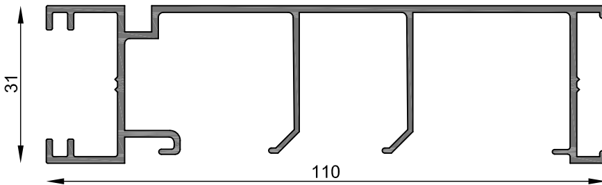
MT-0899 Zócalo Peso estimado: 0.988 Kg/m Largo STD: 6030 mm
