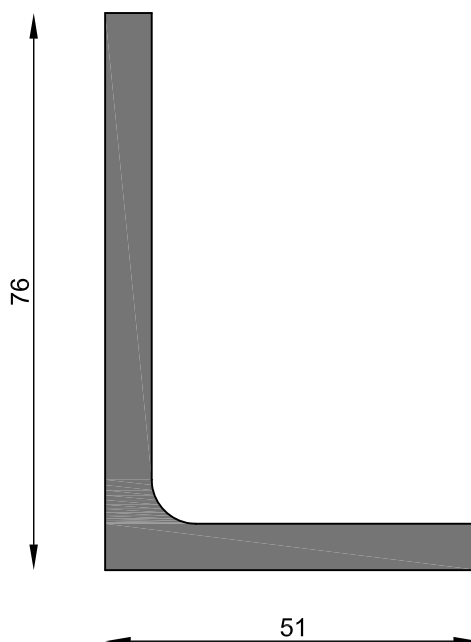
MT-5605 Anclaje inferior de columna ANC 964/966 Peso estimado: 2.087 Kg/m Largo STD: 6030 mm
