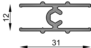
MT-1346 Travesaño intermedio hoja cubre bañera Peso estimado: 0.305 Kg/m Largo STD: 6030 mm
