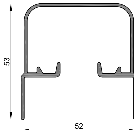
MT-1345 Cabezal cubre bañera Peso estimado: 0.770 Kg/m Largo STD: 6030 mm
