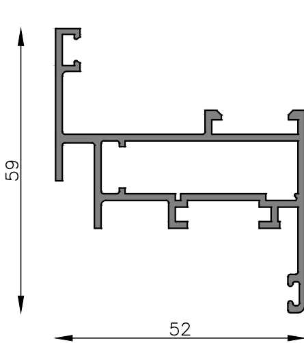
MT-0215 Hoja de abrir doble contacto Peso estimado: 0.861 Kg/m Largo STD: 6150 mm
