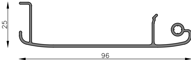
MT-0244 Guía de cortina barro Peso estimado: 0.896 Kg/m Largo STD: 6150 mm
