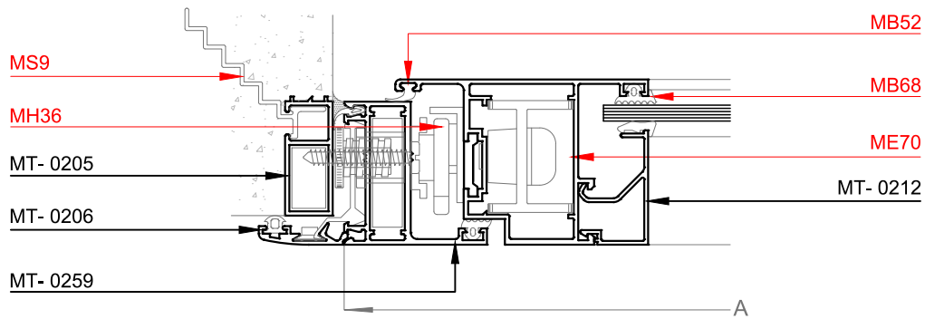
Corte 3-3
