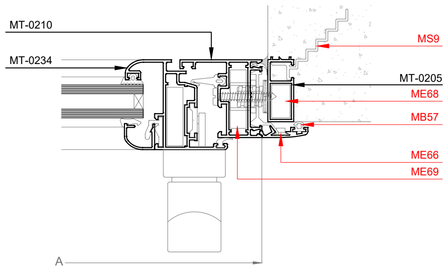
Corte 5"-5"
