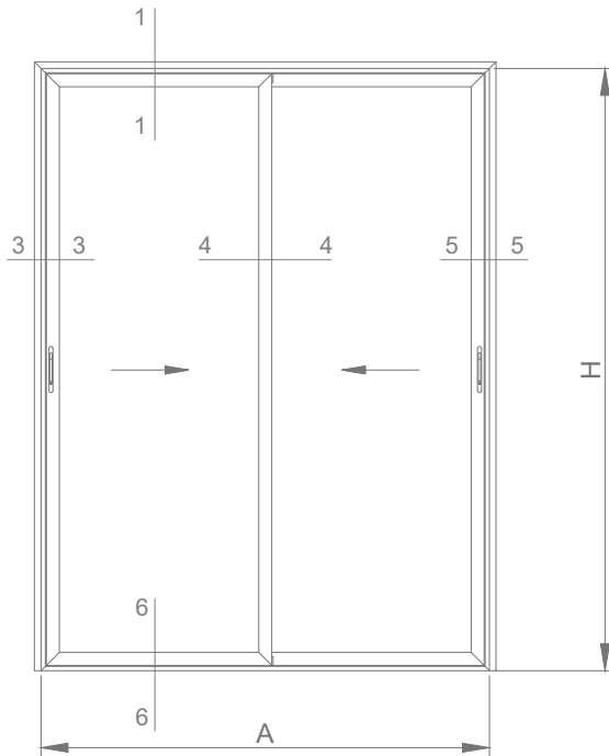
Dimensiones de corte de perfiles
