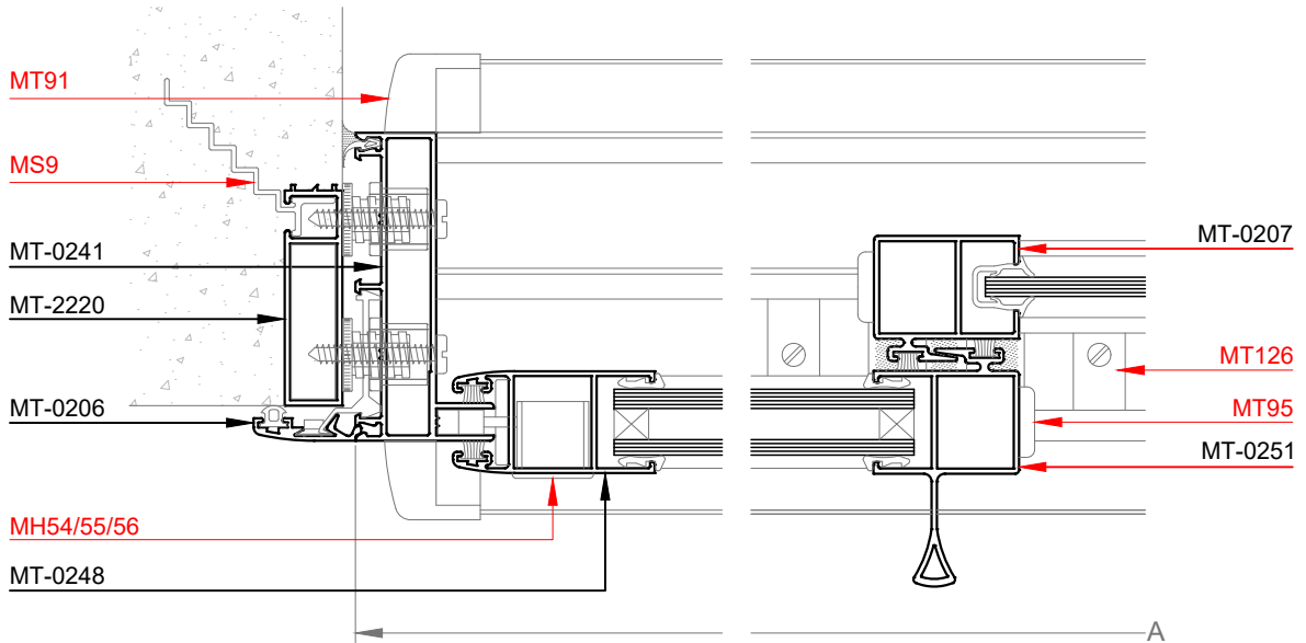
Corte 5-5
