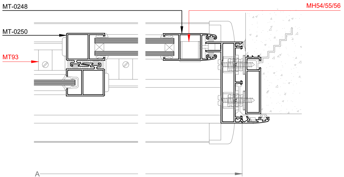
Corte 5-5
