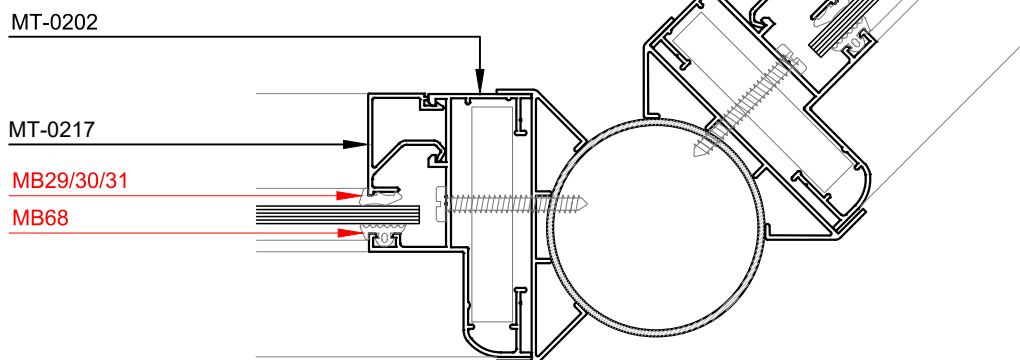
Columna-Apoyo rótula
