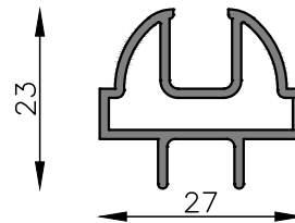
MT-0267 Perimetral de vidrio repartido para corredizas Peso estimado: 0.348 Kg/m Largo STD: 6030 mm
