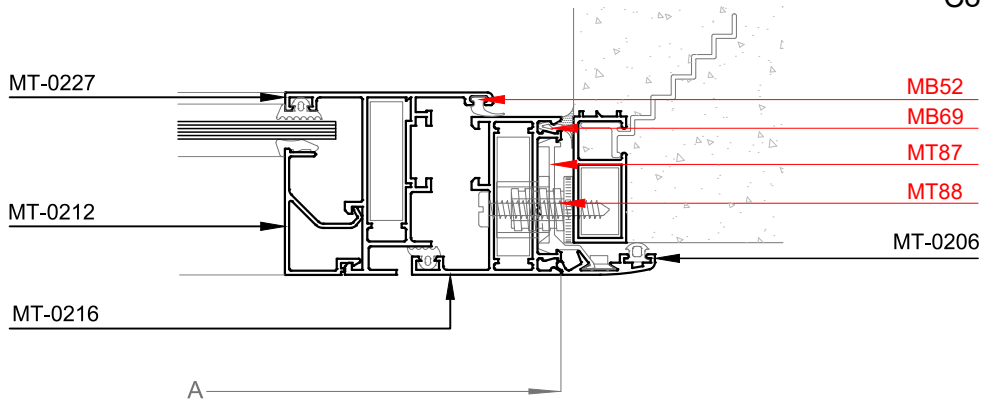
Corte 4-4
