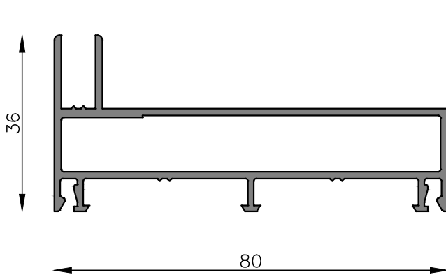
MT-0241 Jamba de marco de tres guías Peso estimado: 0.969 Kg/m Largo STD: 6150 mm
