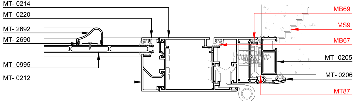
Corte 3-3
