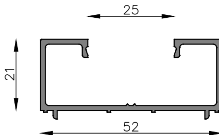
MT-0272 Adaptador para celosía Peso estimado: 0.486 Kg/m Largo STD: 6150 mm
