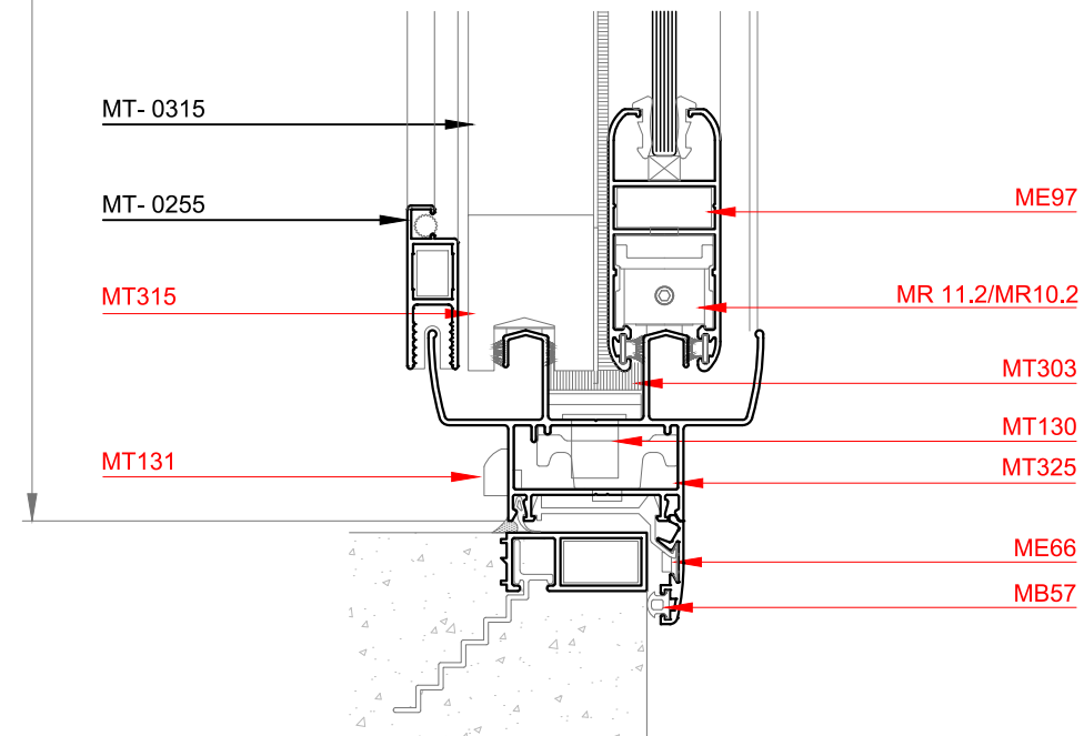
Corte 2-2
