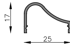
MT-2692 Moldura puerta placa Peso estimado: 0.162 Kg/m Largo STD: 6030 mm
