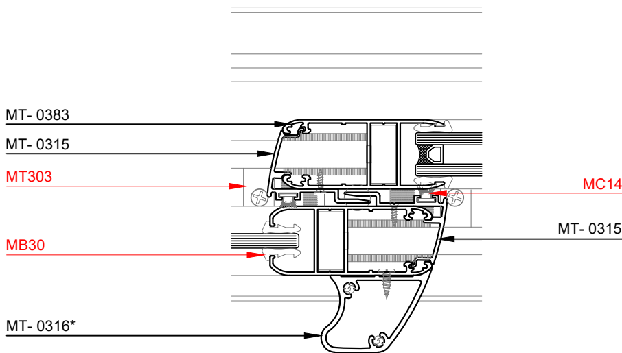
Corte 4-4
