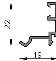
MT-0220 Contra Vidrio exterior puerta de rebatir Peso estimado: 0.176 Kg/m Largo STD: 6030 mm
