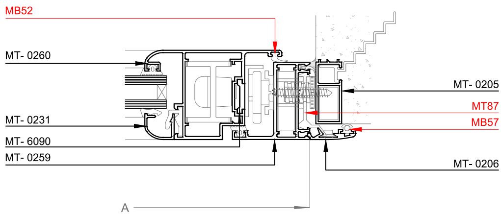
Corte 4'-4'
