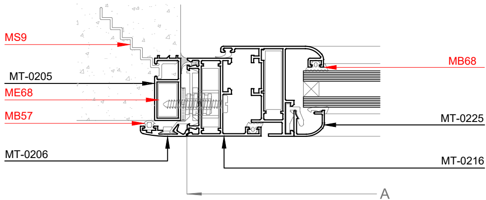
Corte 3-3
