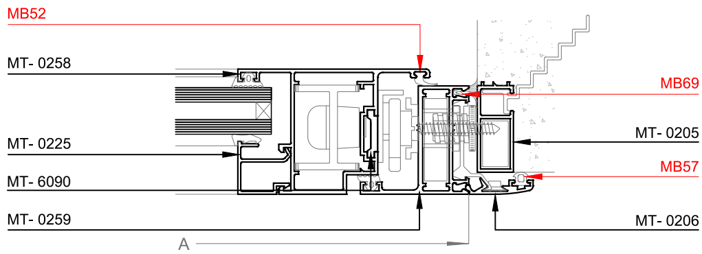
Corte 4-4
