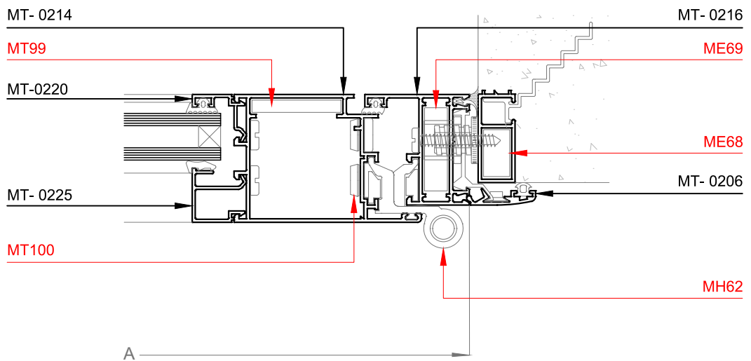
Corte 5-5
