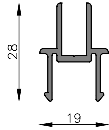
MT-0246 Encuentro central corrediza Peso estimado: 0.292 Kg/m Largo STD: 6030 mm
