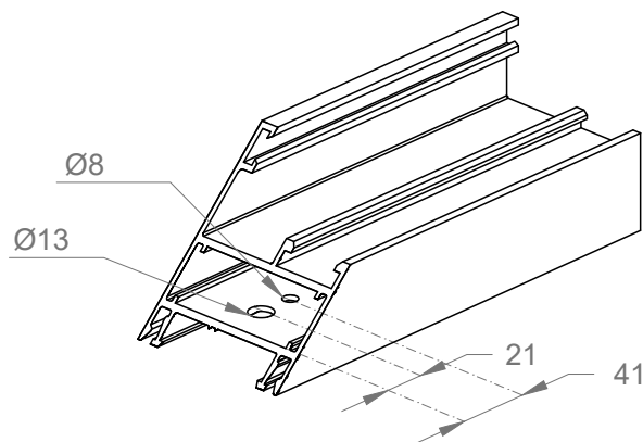
Mecanizado de marco y hoja para escuadras ME69
