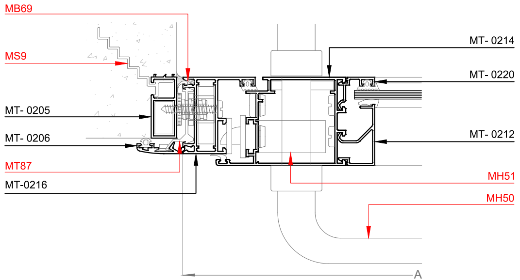
Corte 4-4
