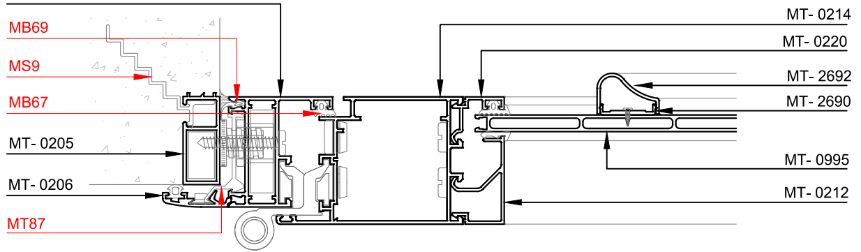
Corte 1-1
