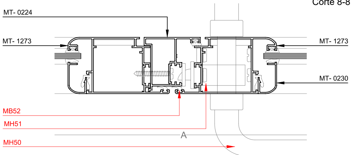
Corte 8-8
