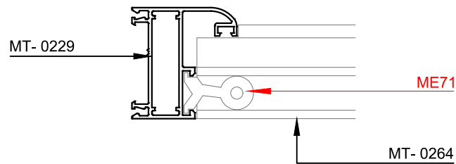
Detalle ensamble con travesaño
