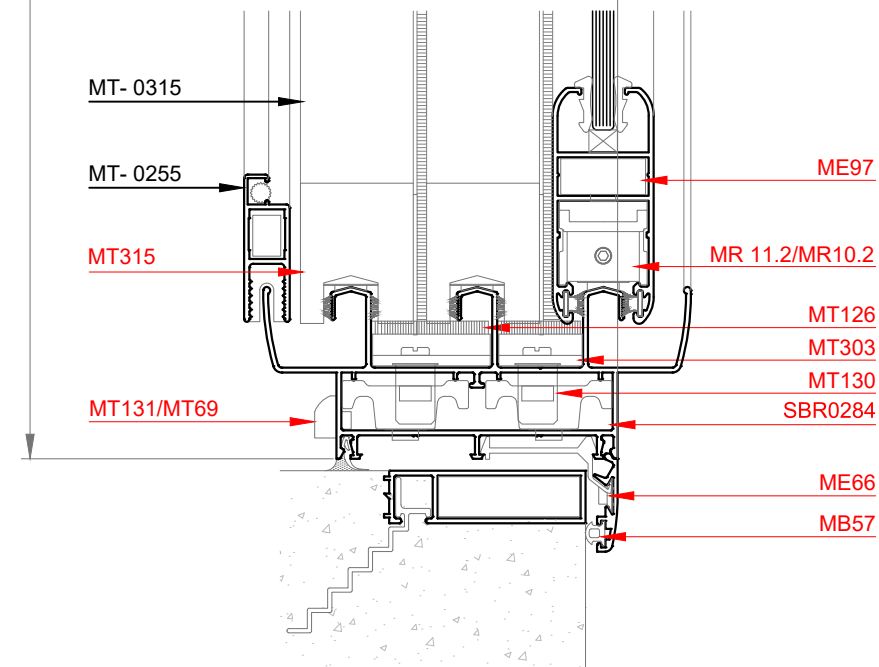
Corte 2-2
