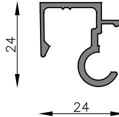
MT-0254 Bisagra tapa cinta Peso estimado: 0.289 Kg/m Largo STD: 6150 mm
