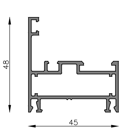
MT-0210 Marco ventana abrir Peso estimado: 0.786 Kg/m Largo STD: 6150 mm
