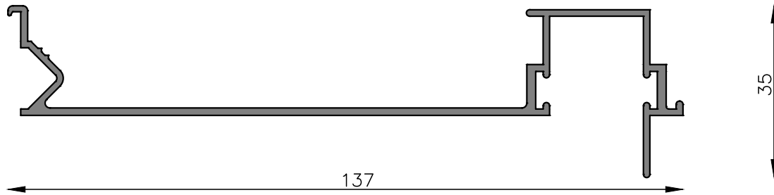
MT-0244 Guía de cortina barro Peso estimado: 0.896 Kg/m Largo STD: 6150 mm
