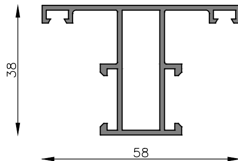
MT-0264 Travesaño paño fijo curvo Peso estimado: 0.713 Kg/m Largo STD: 6030 mm
