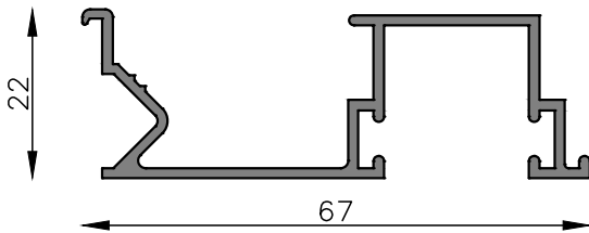
MT-0243 Guía de cortina común Peso estimado: 0.545 Kg/m Largo STD: 6150 mm
