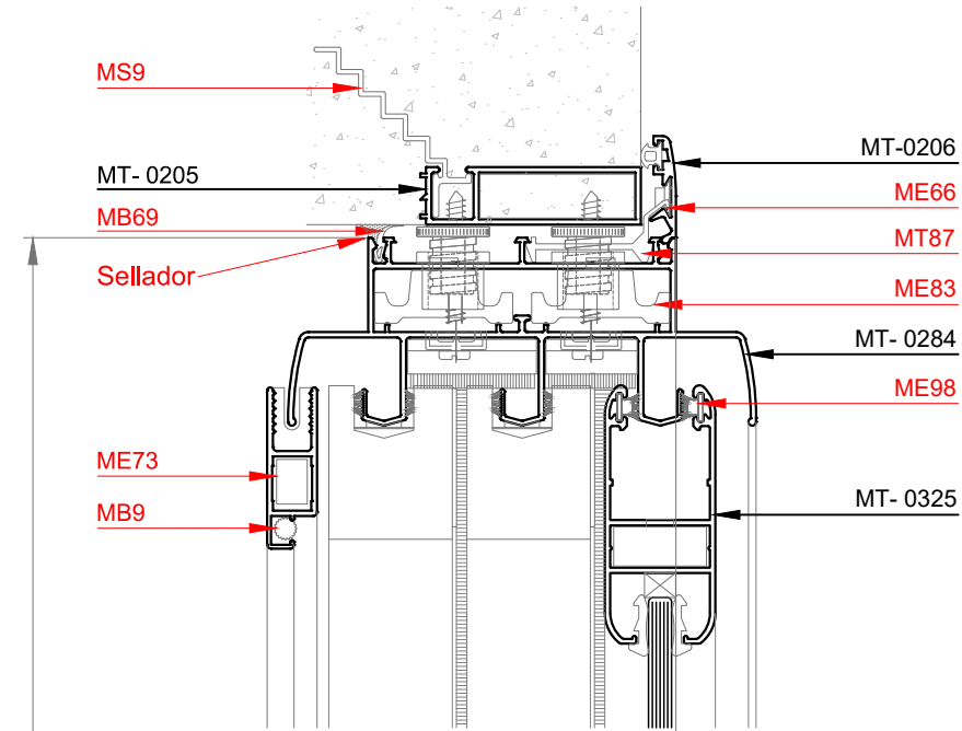
Corte 1-1
