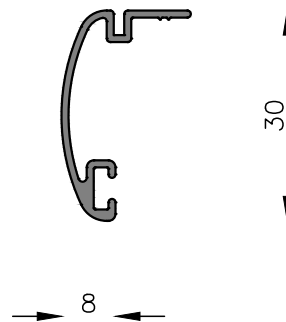
MT-0906 Contramarco Peso estimado: 0.186 Kg/m Largo STD: 6030 mm
