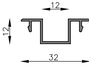
MT-2695 Adaptador hoja regulable Peso estimado: 0.173 Kg/m Largo STD: 6030 mm
